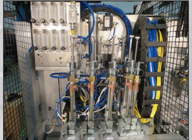
Remachado por aire caliente-herramiental frío
