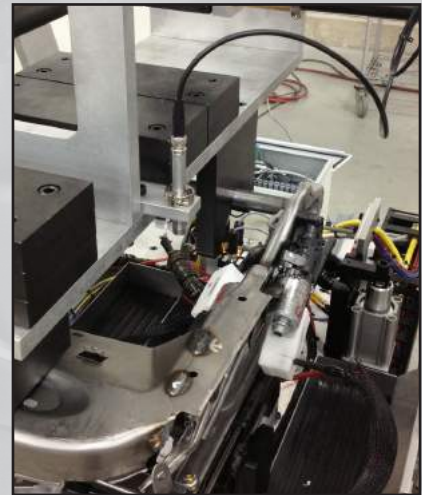
Prueba de movimiento de motores de asientos
