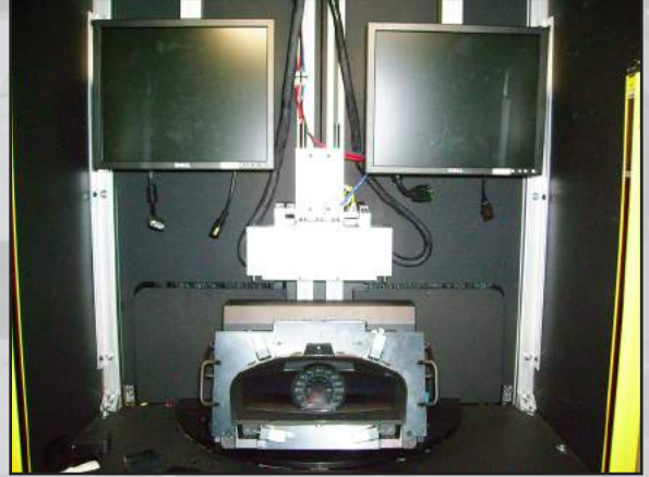
Sistema de visión para verificar pantalla correcta
